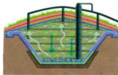
Illustration du captage de biogaz
